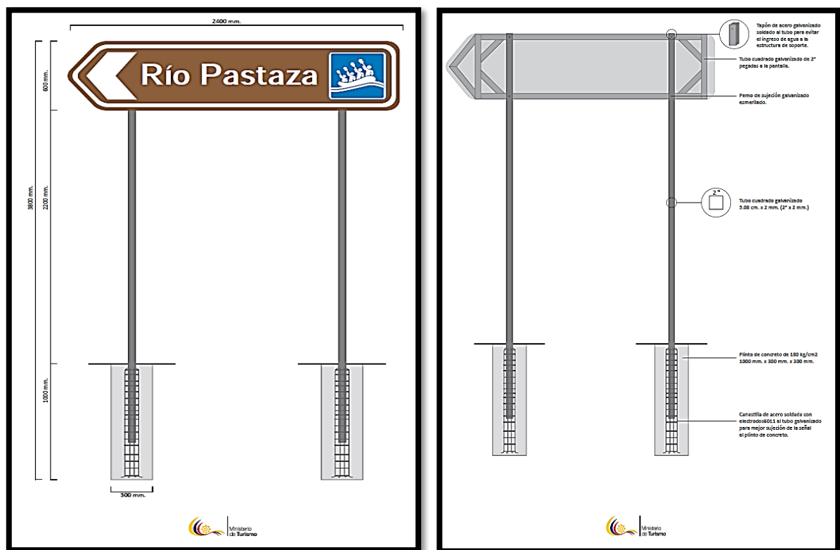
Figura N° 59 Aplicación gráfica: Señal informativa de destino
