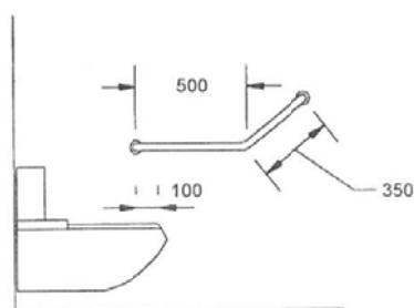
Barra fija tipo 2
