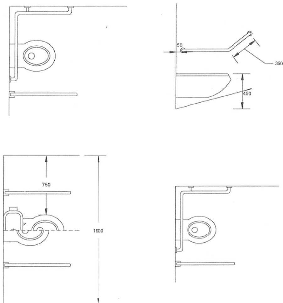
FIGURA 19. Barras de apoyo. Tipos. (Dimensiones en mm)
