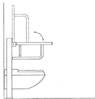
Barra abatible tipo 2
