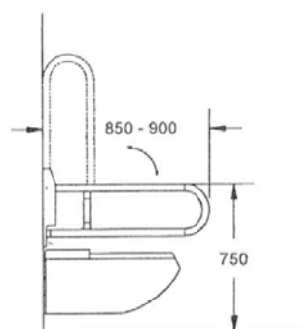
Barra abatible tipo 1
