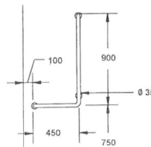
Barra fija tipo 2
