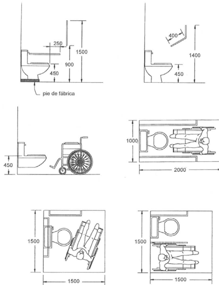
FIGURA 11. Inodoro. Espacio de utilización. (Dimensiones en mm)
