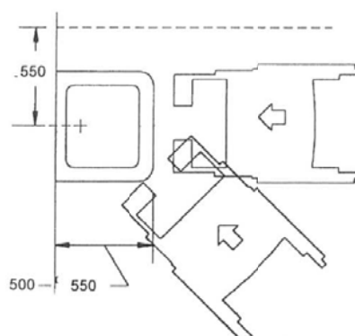
FIGURA 7. Localización del lavabo. (Dimensiones en mm)
