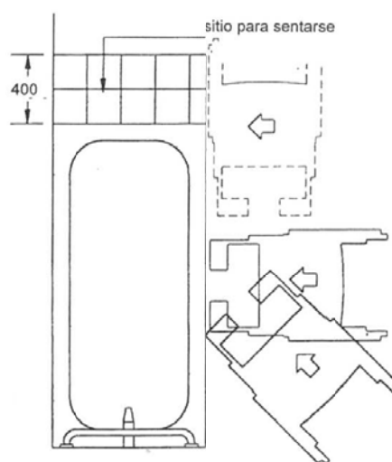
FIGURA 13. Localización de la tina
